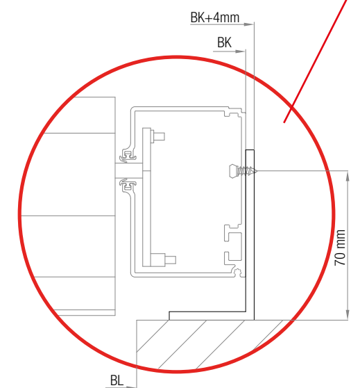
Sezione orizzontale Horizontal section
